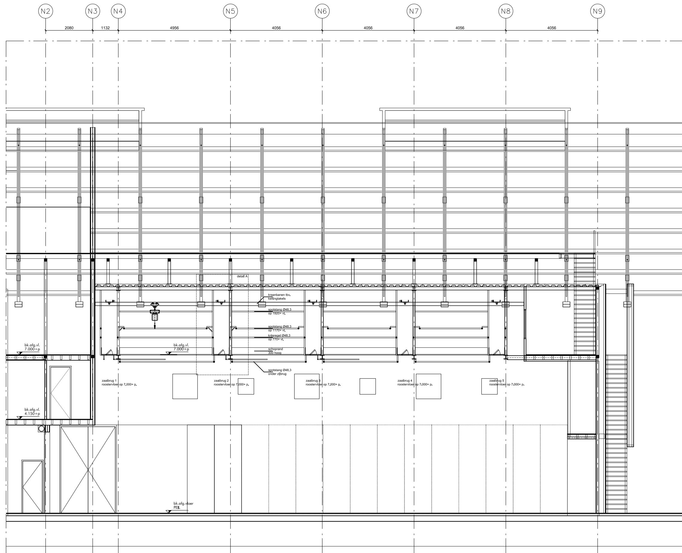
langsdoorsnede
