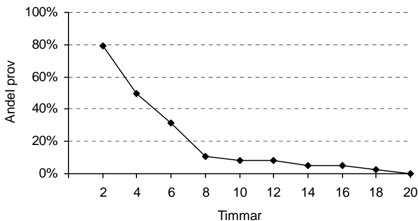
Figur 8. Andel prov där tiden för nedkylning från tillagning tills 8 °C uppnått överskred visst antal timmar.
