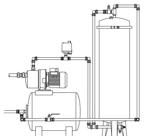
Montering med pumpautomat
