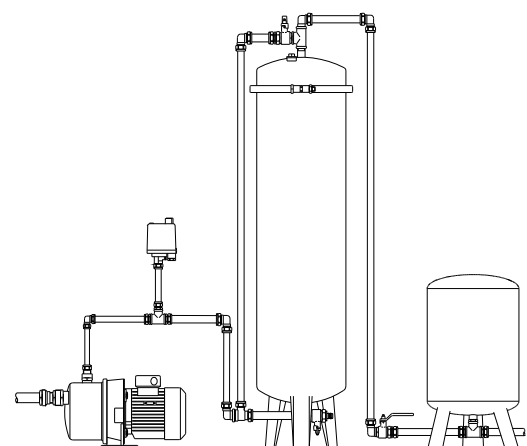
Montering med hydrofor
