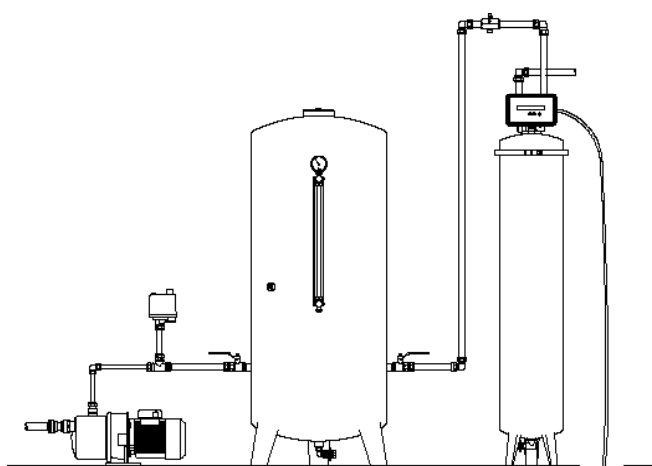
Ferrolite och luftinjektor mot hydrofor
