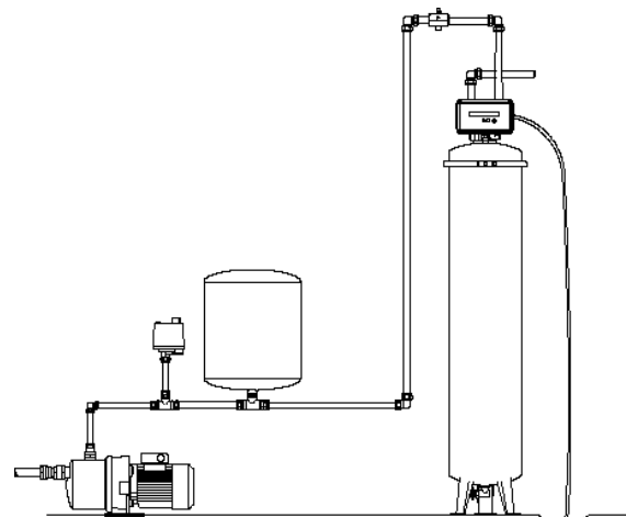
Ferrolite och luftinjektor mot hydropress
