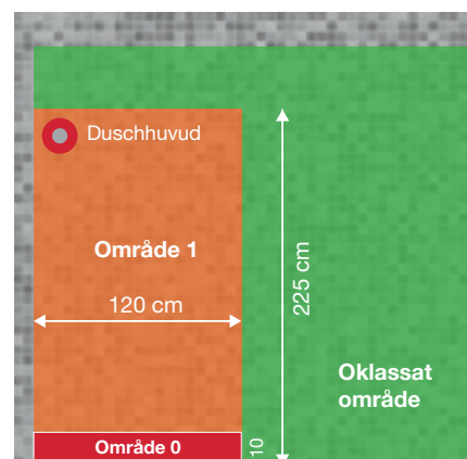
Fig 24. Områdesindelning - Dusch utan kar.
