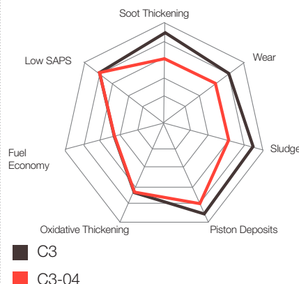
Fig. 2 ACEA C3
