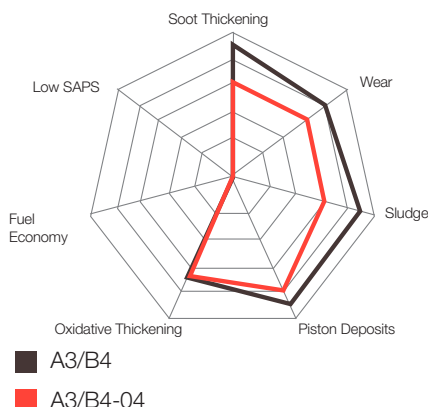
Fig. 1 ACEA A3/B4
