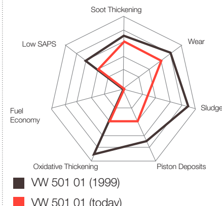
Fig. 3 VW 501 01
