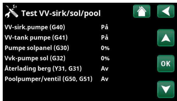
Meny «Avansert/Service/Funksjonstest/VV-sirkulasjon/Sol/Pool».
