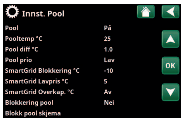
Meny «Avansert/Innstillinger/Pool».
