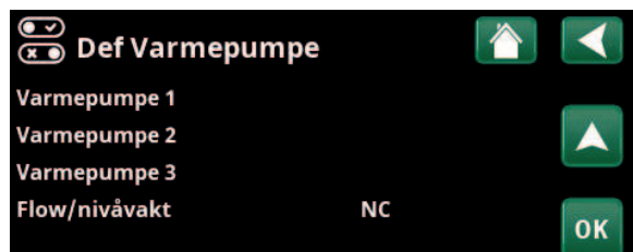
Meny «Avansert/Definere/Varmepumpe».
