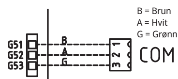
Detaljbilde fra koblingsskjema.
