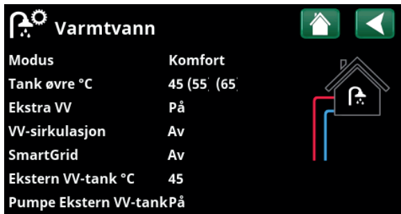
Meny «Driftsinfo/Varmtvann».
