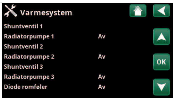
Meny «Avansert/Service/Funksjonstest/Varmesystem».
