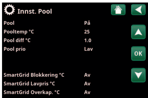
Meny «Avansert/Innstillinger/Pool».
