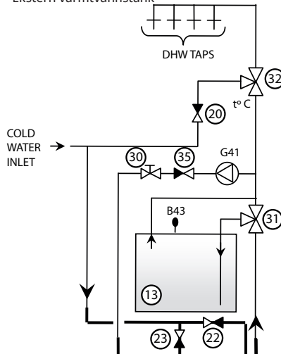
Ekstern varmtvannstank
