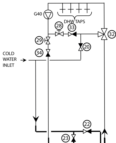
Bilde 1. Varmtvannssirkulasjon
