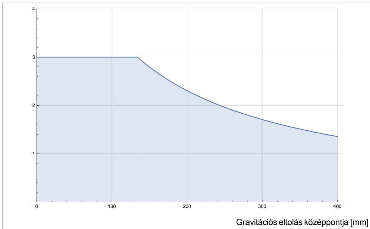
5.3: A maximálisan megengedett hasznos teher és a gravitációs eltolás középpontja közötti kapcsolat.
