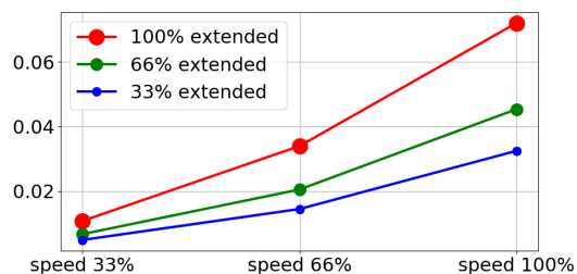
Leállítási távolság méterben a maximális hasznos teher 66%-a esetén
