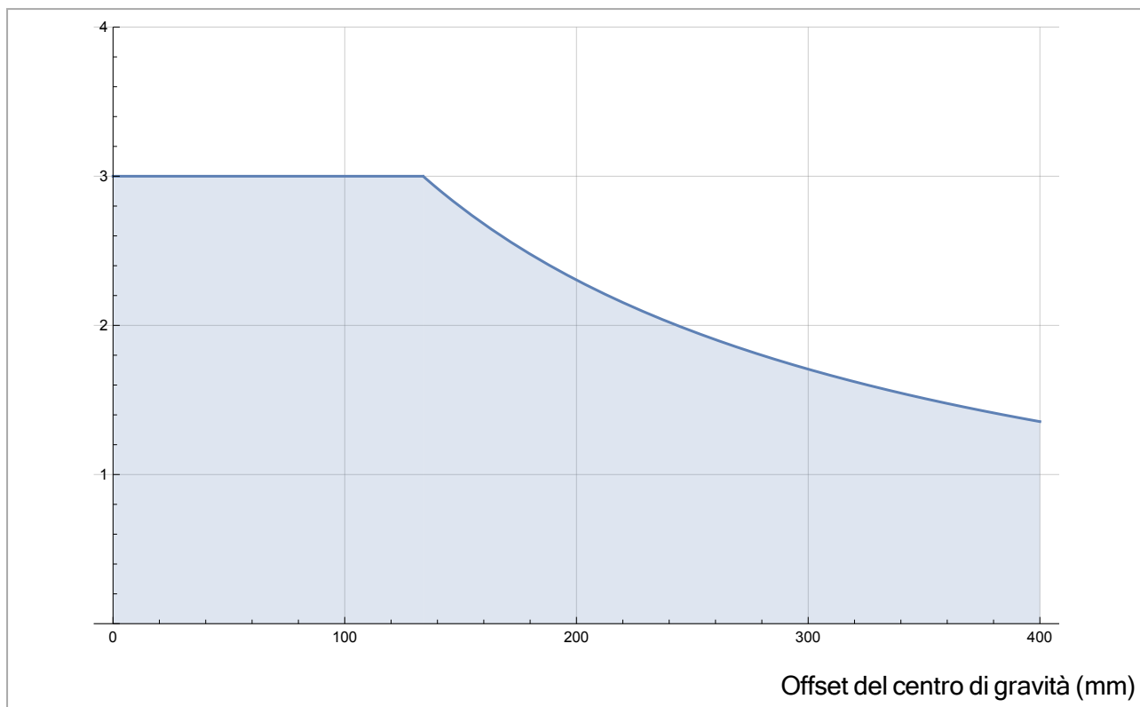
6.3: Rapporto fra il carico utile massimo consentito e l'offset del centro di gravità.
