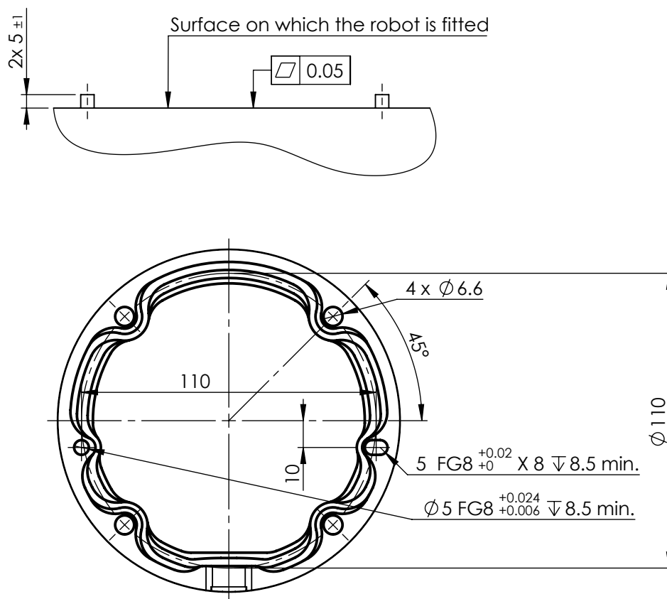
6.1: Fori di montaggio del robot. Utilizzare quattro bulloni M6 . Tutte le misure sono in mm .
