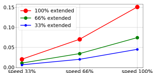
Vzdálenost do zastavení v metrech při 33% maximálního zatížení
