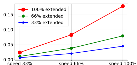
Vzdálenost do zastavení v metrech při 66% maximálního zatížení
