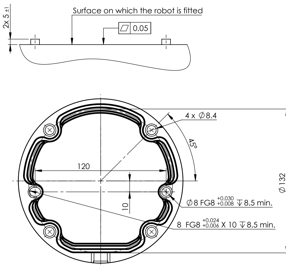
6.1: Otvory pro montáž robota. Použít čtyři M8 šrouby. Všechny míry jsou uvedeny v mm .
