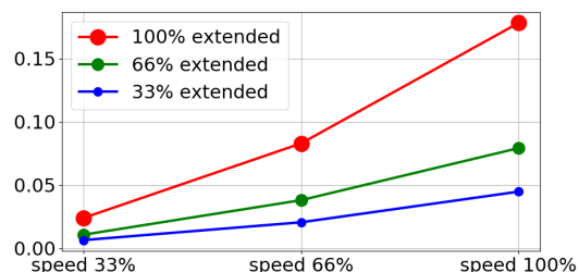
Stoppeavstand i meter for 66 % av maksimal nyttelast
