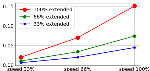
Stoppeavstand i meter for 33 % av maksimal nyttelast
