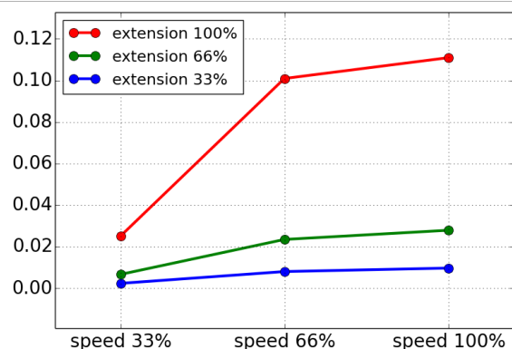
Stopafstand i meter for 66 % af maksimal nyttelast
