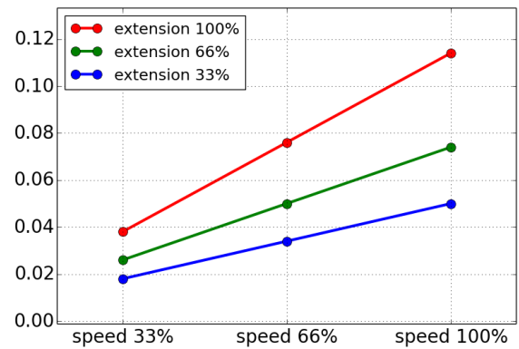
Stoptid i sekunder for 66 % af maksimal nyttelast
