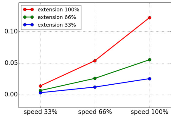
Stopafstand i meter for maksimal nyttelast
