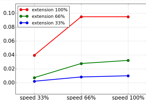
Stopafstand i meter for maksimal nyttelast
