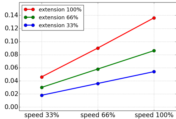
Stoptid i sekunder for maksimal nyttelast
