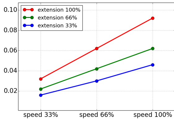
Stoptid i sekunder for 33 % af maksimal nyttelast
