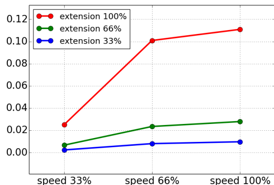
Vzdialenosť zastavenia v metroch pri 66 % maximálneho zaťaženia
