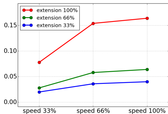
Čas zastavenia v sekundách pri 66 % maximálneho zaťaženia
