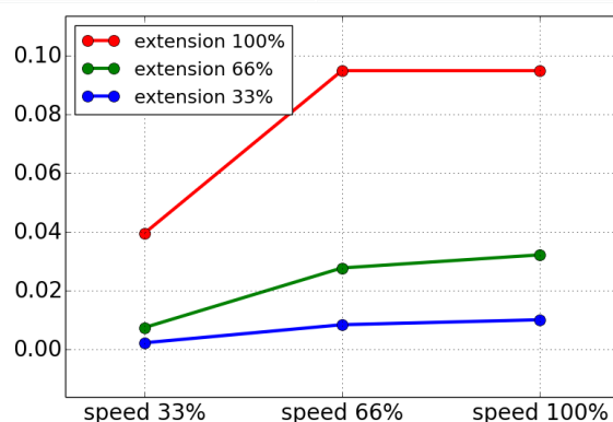
Vzdialenosť zastavenia v metroch pre maximálne zaťaženie
