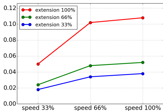
Čas zastavenia v sekundách pri 33 % maximálneho zaťaženia
