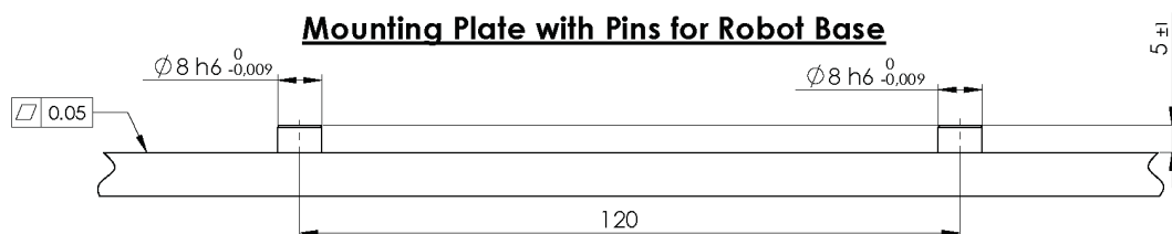
6.1: Huller til montering af robotten. Brug fire M8 bolte. Alle mål er i mm .
