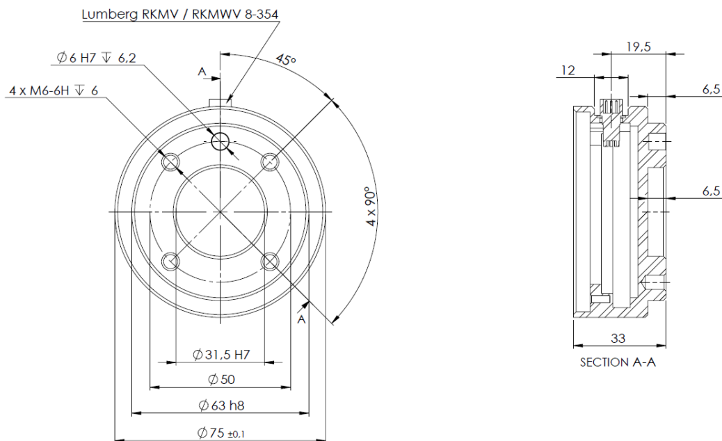
6.2: Brida de salida de la herramienta, ISO 9409-1-50-4-M6. Aquí es donde se monta la herramienta, en la punta del robot. Todas las medidas están en mm.
