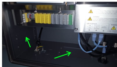
18.2: Schnittstellenbestückung in der Control-Box
