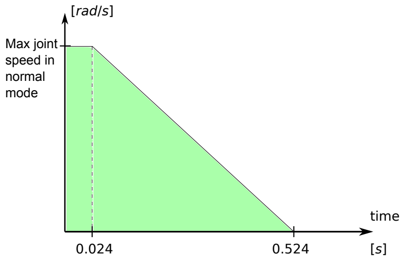
4.2: Der grüne Bereich unterhalb der Rampe markiert die zulässigen Geschwindigkeiten für ein Gelenk beim Bremsen. Zum Zeitpunkt 0 wird ein Ereignis (Notabschaltung oder Schutzstopp) am Sicherheitsprozessor erfasst. Der Abbremsvorgang beginnt nach 24 ms.
