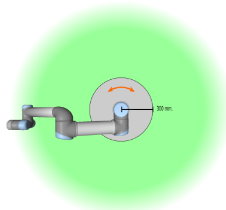
4.1: Bestimmte Teile des Wirkungsbereichs bergen aufgrund der physikalischen Eigenschaften des Roboterarms erhöhte Quetschgefahr. Dazu gehört bei radialen Bewegungen das Handgelenk 1, wenn es mindestens 1300 mm vom Basisflansch des Roboters entfernt ist. Der andere Teil befindet sich bei Tangentialbewegung innerhalb von 300 mm vom Basisflansch des Roboters.
