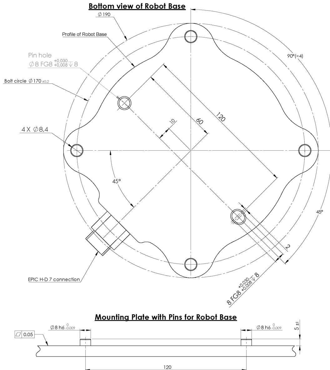
6.1: Löcher zur Montage des Roboters. Verwenden Sie vier M8 Schrauben. Alle Maßangaben sind in mm.
