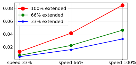
Distanza di arresto in metri per il carico utile massimo di 3 kg
