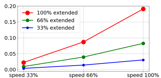
Stopafstand in meters bij 66% van 10 kg
