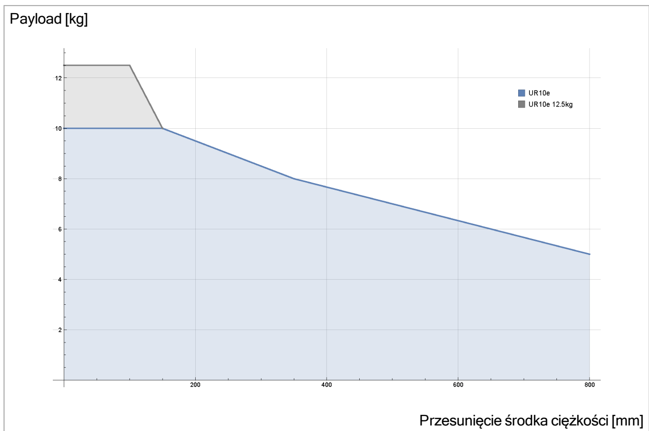
6.3: Relacja między maksymalnym dopuszczalnym obciążeniem a przesunięciem środka ciężkości.
