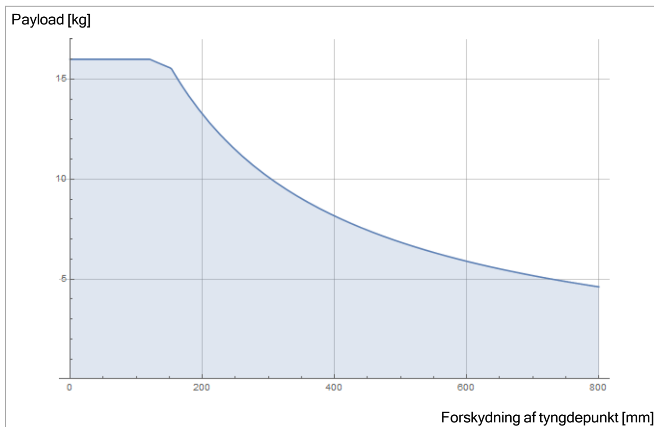
6.3: Forholdet mellem den maksimalt tilladte nyttelast og forskydningen af tyngdepunktet.
