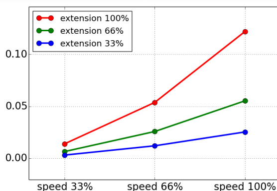
Stopafstand i meter for maksimal nyttelast for 16 kg
