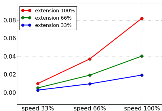
A 0. illesztés (ALAP) leállási távolsága
