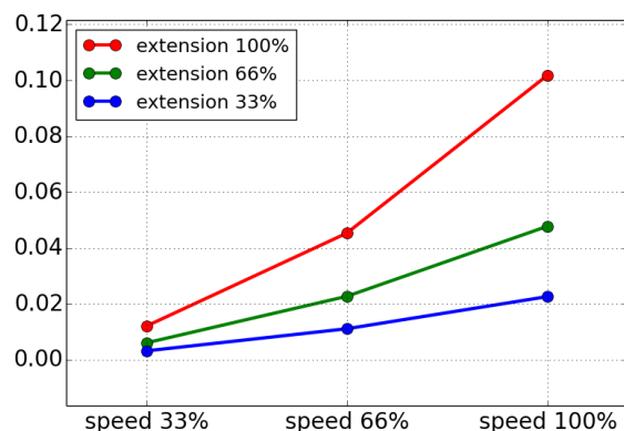
A 0. illesztés (ALAP) leállási távolsága
