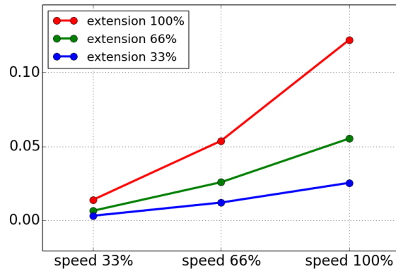
16kg ağırlığının %33'ü için metre cinsinden durdurma mesafesi
