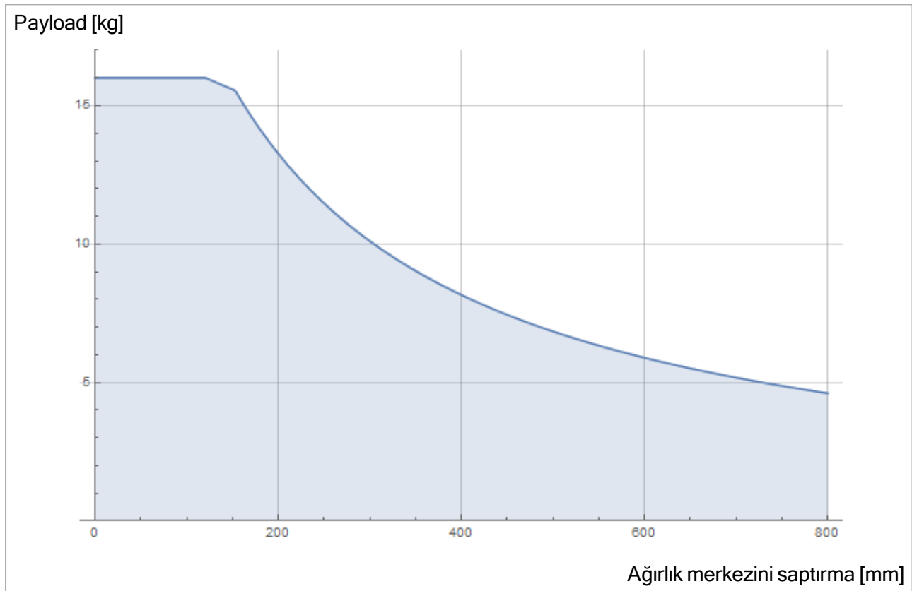
6.3: İzin verilen maksimum taşıma kapasitesiyle ağırlık merkezini ofseti arasındaki ilişki.
