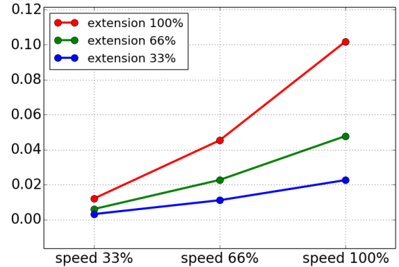
16kg ağırlığının %66'sı için metre cinsinden durdurma mesafesi
