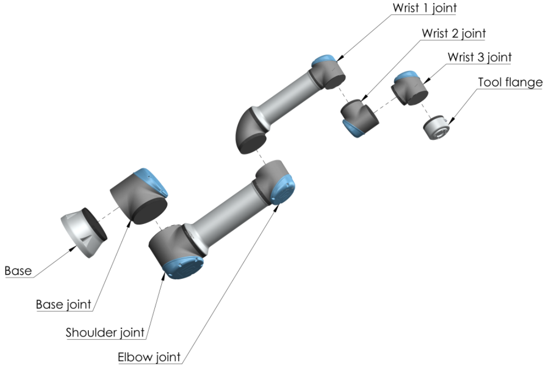
2.1: Robot Kolunun eklemleri, tabanı ve alet flanşı.
