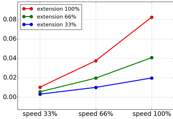
16kg ağırlığının %33'ü için metre cinsinden durdurma mesafesi
