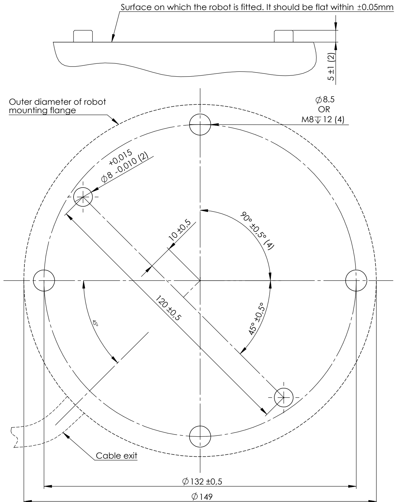
Figur 3.1: Huller til montering af robotten. Brug fire M8-bolte. Alle mål er i mm.
