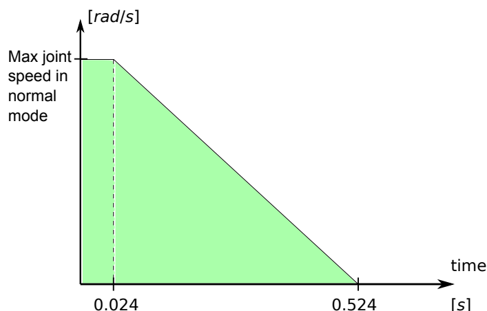
Rysunek 5.2: Zielone pole poniżej nachylenia odpowiada dopuszczalnym prędkościom przegubu podczas hamowania. W chwili 0 procesor bezpieczeństwa wykrywa zdarzenie (zatrzymanie awaryjne lub przez zabezpieczenie). Wyhamowywanie rozpoczyna się po 24 ms.
