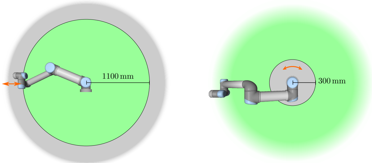
Figure 5.1: 작업영역의 특정영역은 로봇팔의 물리적 특성 때문에 집히는 위험을 주의해야 한다. 리스트 1 조인트가 로봇베이스로부터 최소한 1100 mm 거리인 경우에 한영역이 방사형 동작을 위해 정의된다. 접선방향으로 움직이는 경우, 다른영역은 로봇베이스로부터 300 mm 거리내에 있다.
