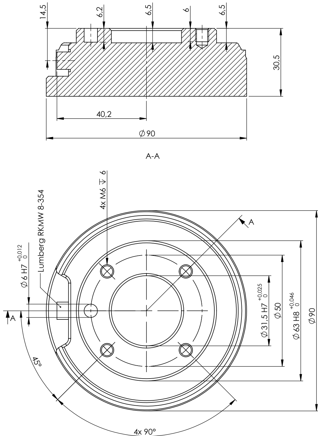
Figure 3.2: 토크출력플렌지, ISO 9409-1-50-4-M6. 여기가 로봇끝에서 토크를 마운트하는 위치이다. 모든 측정 단위는 mm 이다.
