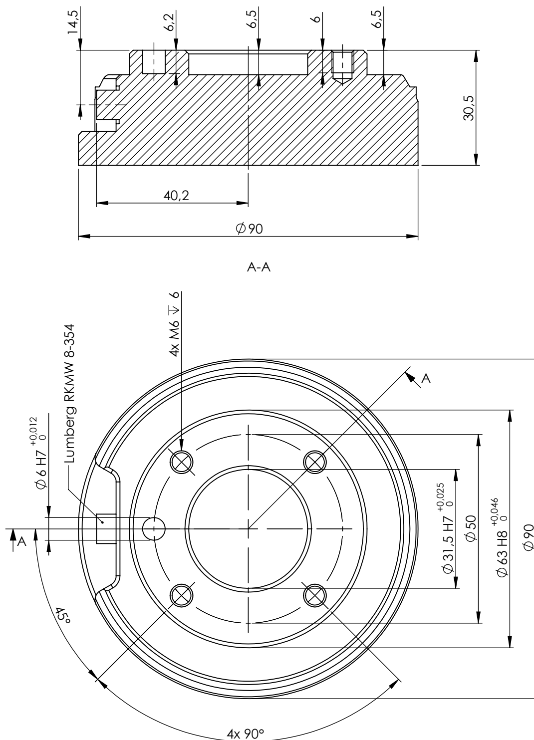
Rysunek 3.2: Kołnierz wyjściowy narzędzia, ISO 9409-1-50-4-M6. Jest to miejsce montażu narzędzia na końcu robota. Wszystkie wymiary są podane w mm.
