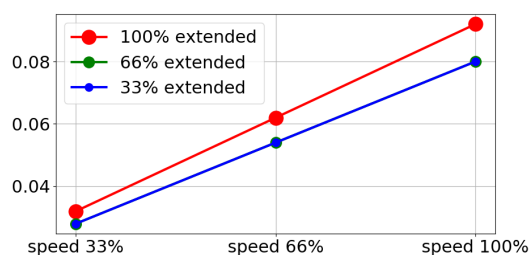
载荷为 3kg 的 66% 时的停止时间(秒)
