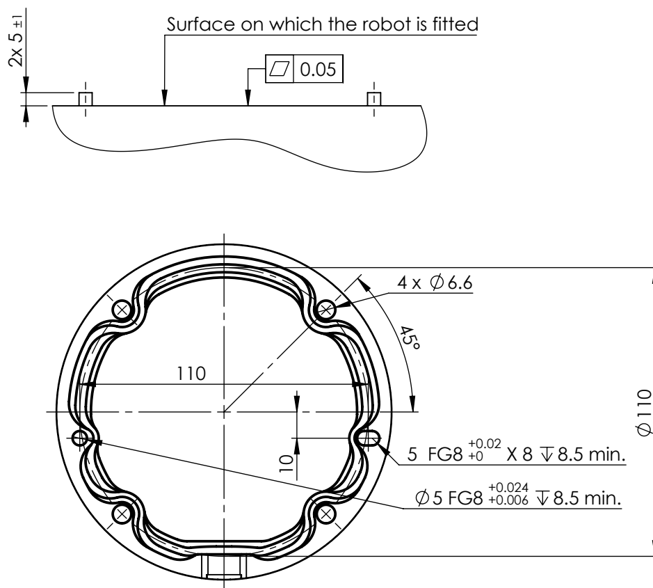
5.1 : 机器人安装孔。使用四颗 M6 螺栓。所有测量值均以 mm 为单位。
