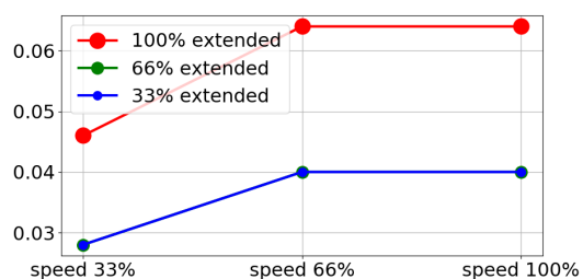
载荷为 3kg 的 33% 时的停止时间(秒)
