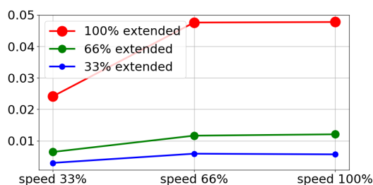
载荷为最大载荷 3kg 时的停止距离(米)
