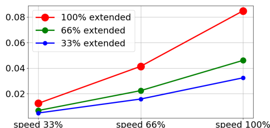
载荷为最大载荷 3kg 时的停止距离(米)
