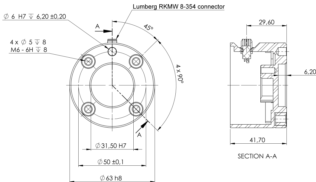
5.2: Výstupná nástrojová príruha (ISO 9409-1-50-4-M6) sa nachádza na mieste, kde je nástroj primontovaný k špičke robota. Všetky rozmery sú v mm.
