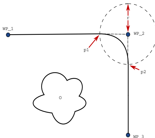
23.3: Zatáčka okolo ( WP\_2 ) s polomerom r , úvodná poloha zatáčania v p1 a koncová poloha zatáčania v p2 . ( O ) je prekážka.
