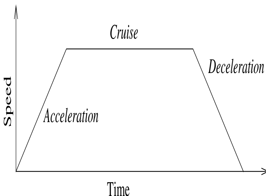
23.1: Rýchlostný profil pohybu. Krivka je rozdelená do troch úsekov: zrýchlenie, rovnomerný pohyb a spomalenie. Rýchlosť vo fáze rovnomerného pohybu je daná nastavením rýchlosti pohybu, zatiaľ čo rýchlosť vo fáze zrýchlenia a spomalenia je daná parametrom zrýchlenia.
