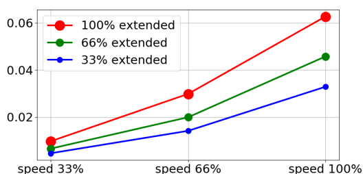
Vzdialenosť zastavenia pre 33 % z 3 kg
