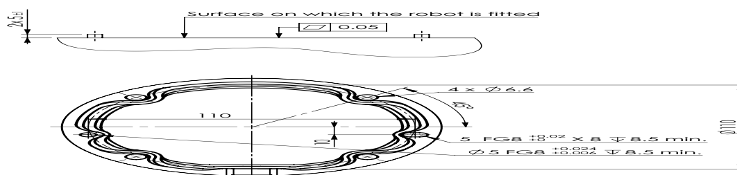
5.1: Otvory na montáž robota. Použite M6 skrutky. Všetky rozmery sú v mm.
