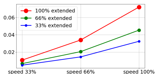
Vzdialenosť zastavenia pre 66 % z 3 kg
