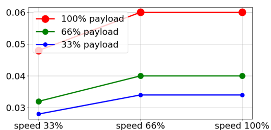
全有効荷重に対する停止時間 (秒)
