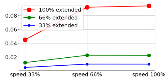
5kg の 66% に対する停止距離 (メートル)
