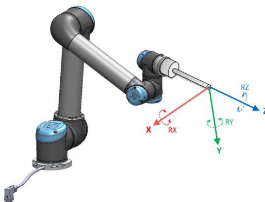
CF :24.2: ツール (TCP) のフィーチャー
