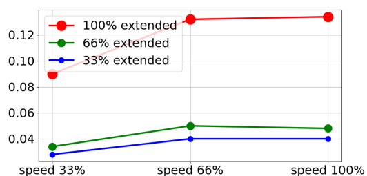
5kg の 66% に対する停止時間 (秒)
