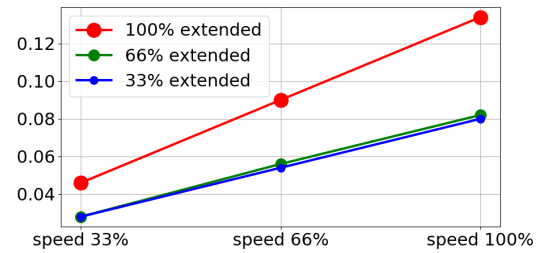
5kg の 66% に対する停止時間 (秒)
