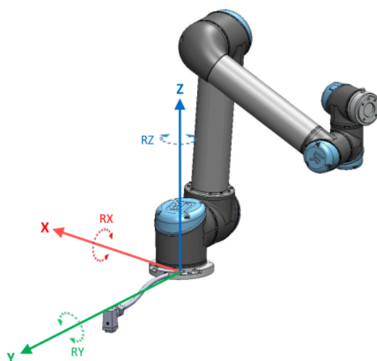
CF :24.1: ベースのフィーチャー
