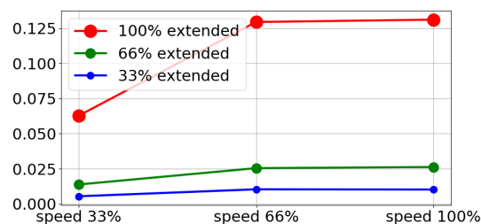
5kg の最大有効荷重に対する停止距離 (メートル)
