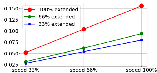
5kg の最大有効荷重に対する停止時間 (秒)
