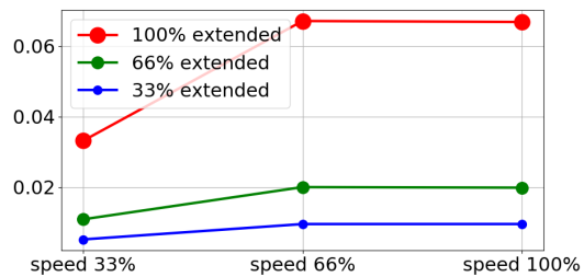
5kg の 33% に対する停止距離 (メートル)
