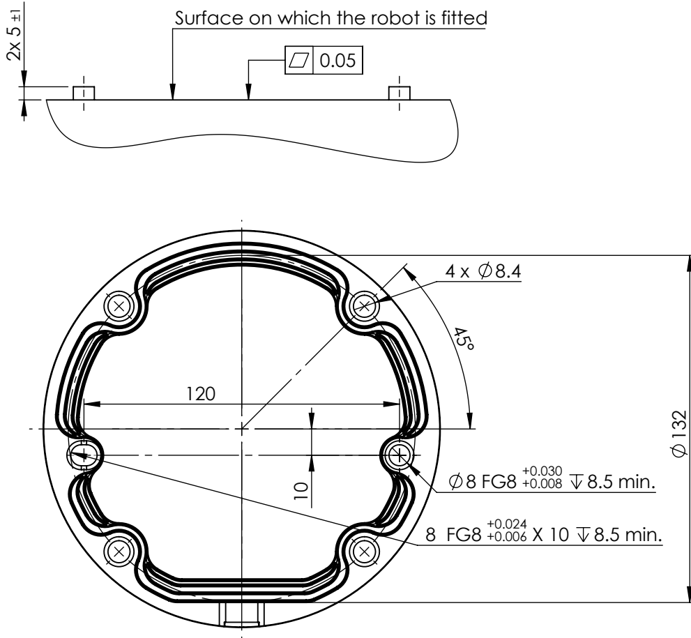
5.1: Robotun montaj delikleri. Dört M8 cıvata kullanın. Bütün ölçüler mm cinsindendir.
