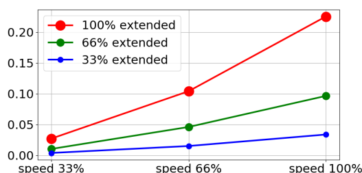
Vzdialenosť zastavenia pre maximálne zaťaženie 10 kg
