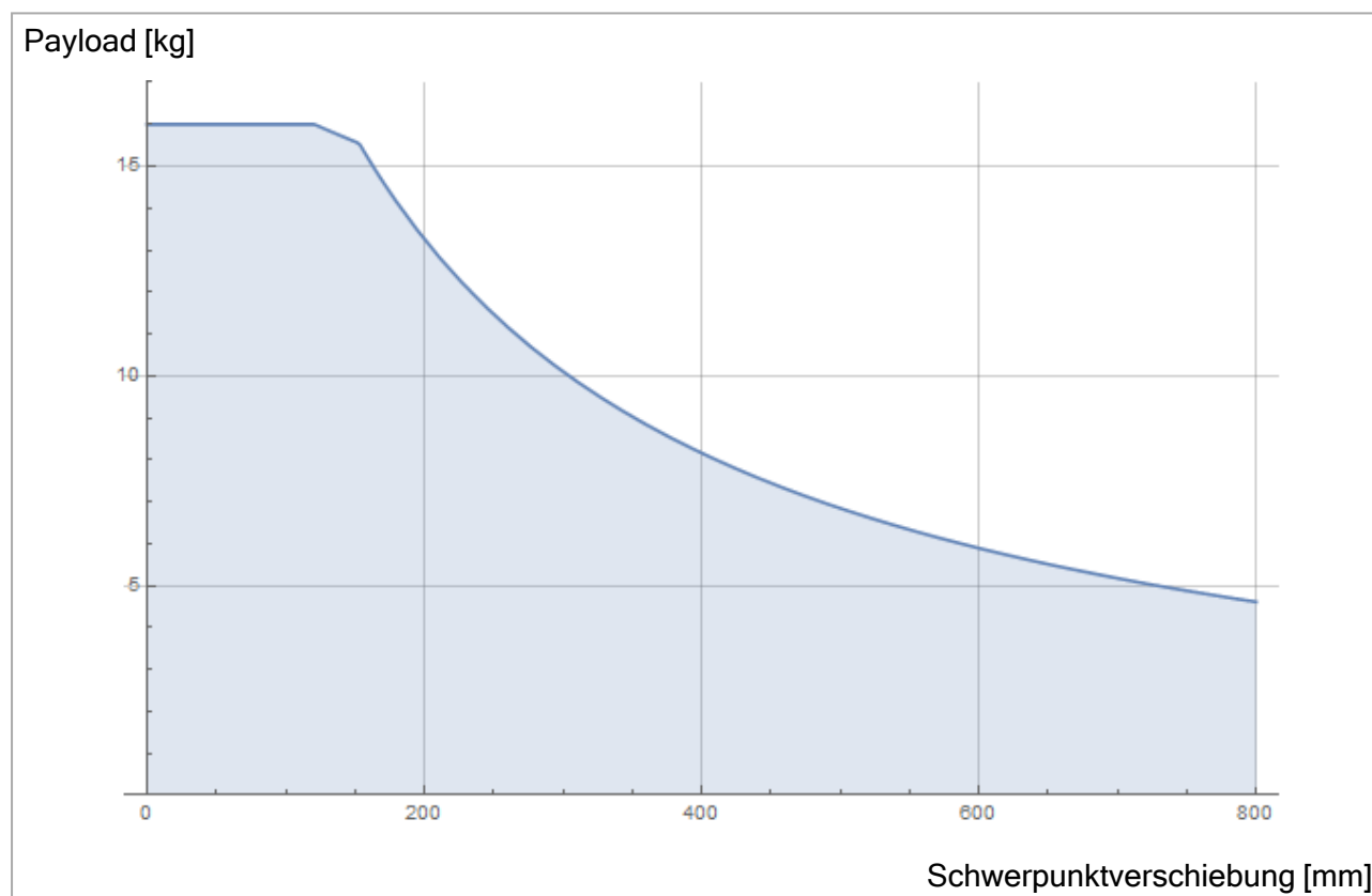
5.3: Beziehung zwischen der Nennnutzlast und der Schwerpunktverschiebung.
