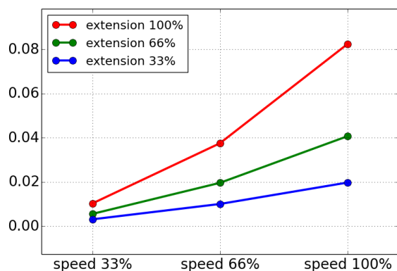
Odległość zatrzymania dla przegubu 0 (PODSTAWA)
