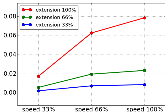
Odległość zatrzymania w metrach dla 33% z 16 kg
