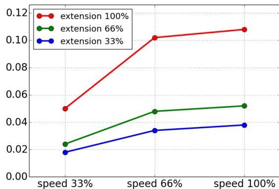
Czas zatrzymania w sekundach dla 33% z 16 kg
