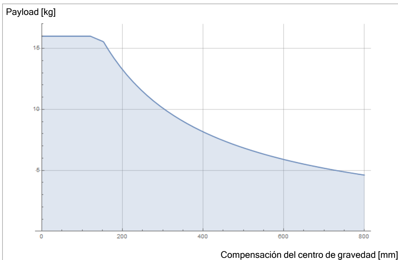
5.3: La relación entre la carga útil nominal y la compensación del centro de gravedad.
