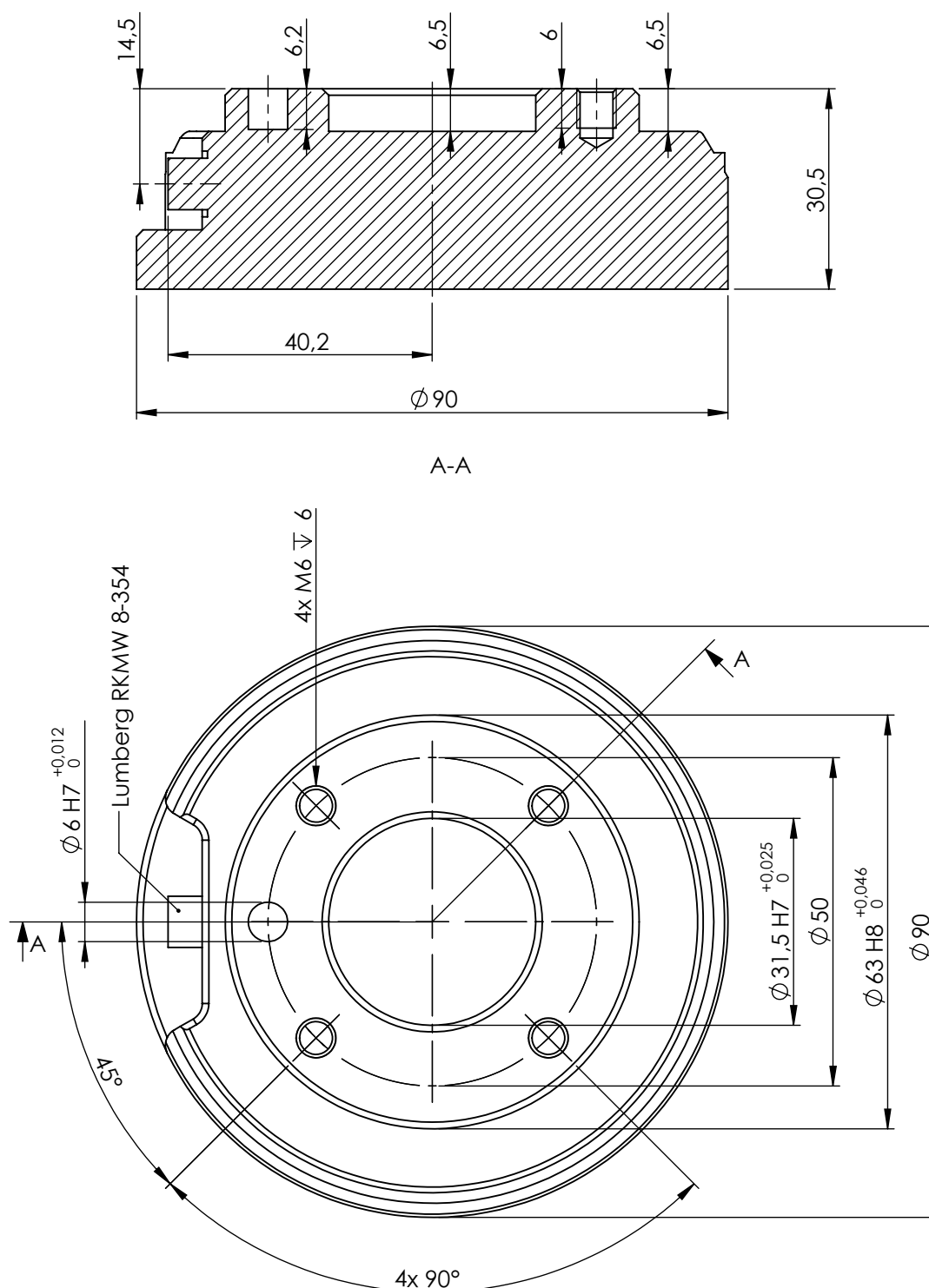
Figur 3.2: Værktøjsoutputflangen, ISO 9409-1-50-4-M6. Det er her, værktøjet monteres på robotten. Alle mål er i mm.
