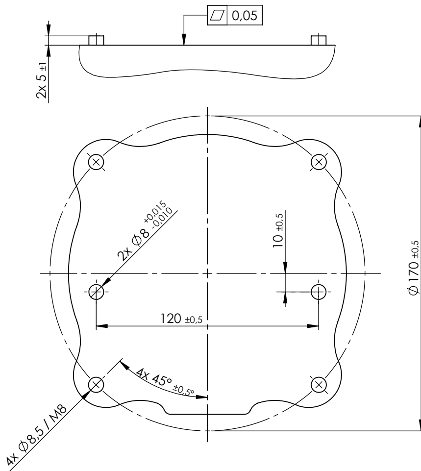
Abbildung 3.1: Löcher zur Montage des Roboters. Verwenden Sie vier M8-Schrauben. Alle Maßangaben sind in mm.
