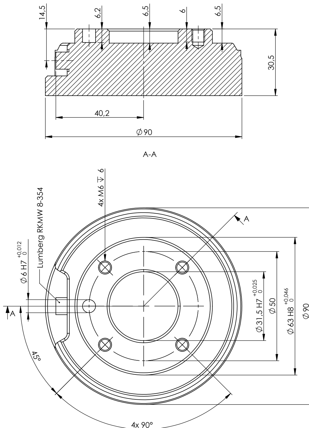
Figura 3.2: La flangia di uscita dell'utensile, ISO 9409-1-50-4-M6. Qui viene montato l'utensile alla sommità del robot. Tutte le misure sono in mm.
