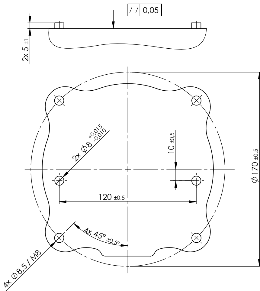
Рис. 3.1: Отверстия для монтажа робота. Используются четыре болта M8. Все измерения приведены в мм.
