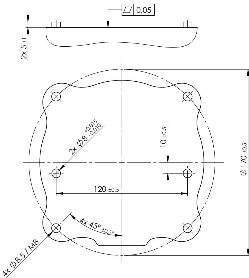
Obr. 3.1: Otvory na montáž robota. Použite štyri skrutky M8. Všetky merania sú v mm.
