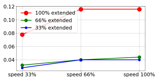
3kg の最大有効荷重に対する停止時間 (秒)
