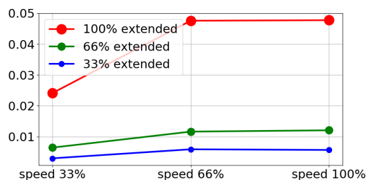
3kg の最大有効荷重に対する停止距離 (メートル)
