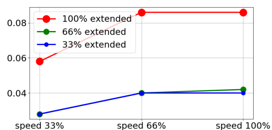
3kg の 66% に対する停止時間 (秒)
