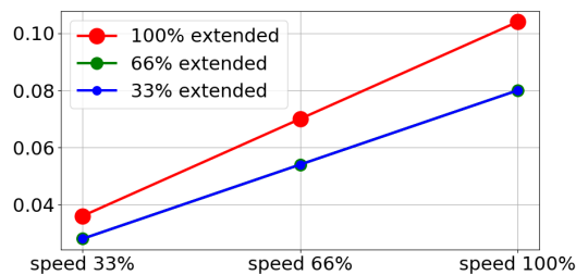
3kg の最大有効荷重に対する停止時間 (秒)
