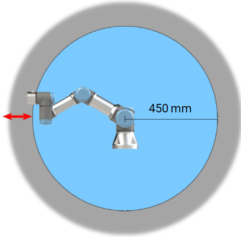
4.1: Robot kolunun fiziksel özelliklerinden dolayı, bazı çalışma alanlarına sıkıştırma tehlikeleriyle ilgili olarak dikkat edilmesi gerekir. Bilek 1 eklemiyle robot tabanı arasında en az 450 mm olduğunda, radyal hareketler için bir alan (sol) tanımlanır. Diğer (sağdaki) alan, teğet hareket ederken robotun tabanının 200 mm yakınındadır.
