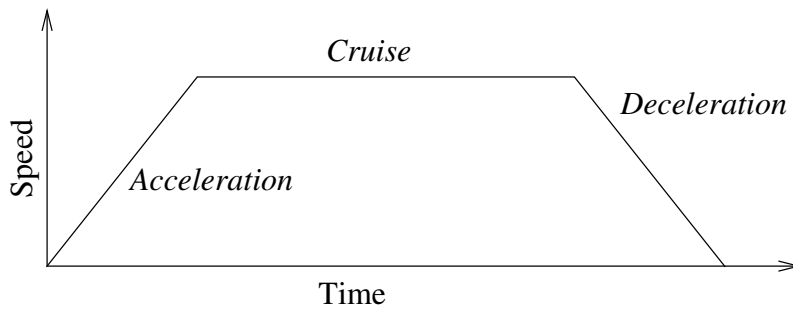
23.1: Bir hareketin hız profili. Eğri, üç kesime ayrılır: ivme, seyir ve yavaşlama. Seyir aşamasının seviyesi, hareketin hız ayarıyla belirlenirken, hızlanma ve yavaşlama aşamalarının dikliği, hızlanma parametresiyle belirlenir.
