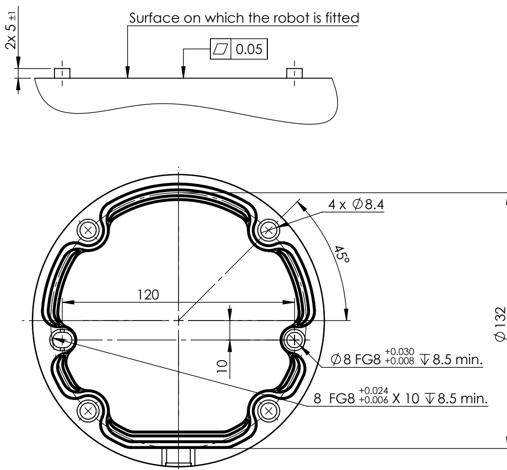
5.1: Hull for montering av roboten. Bruk fire M8 bolter. Alle mål er i mm .
