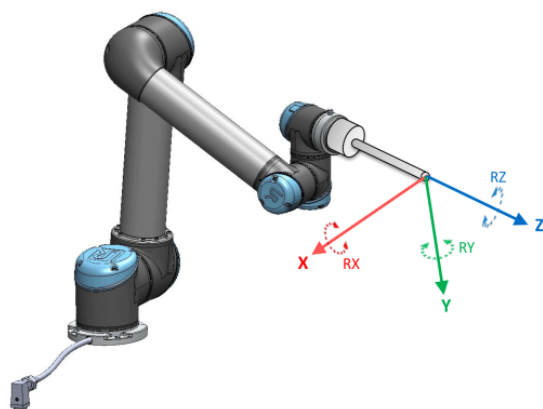
24.2: Verktøyfunksjon (TCP)
