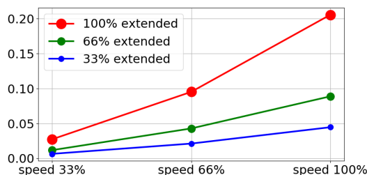
Odległość zatrzymania w metrach dla obciążenia maksymalnego 5 kg
