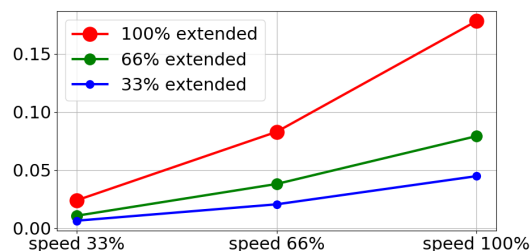
Odległość zatrzymania w metrach dla 66% z 5 kg
