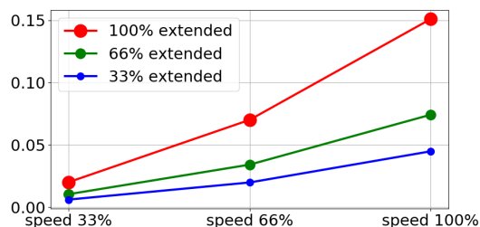
Odległość zatrzymania w metrach dla 33% z 5 kg
