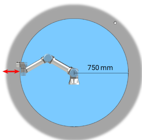
4.1: Zaradi fizičnih značilnosti robotove roke določena delovna območja terjajo pozornost na tveganje stiskanja. Eno območje (levo) je določeno za radialne premike, ko je člen zapestje 1 vsaj 750 mm od osnove robota. Drugo območje (desno) je znotraj 200 mm osnove robota, pri tangentnem premikanju.
