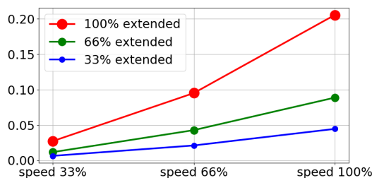
Razdalja ustavljanja v metrih za maksimalno obremenitev 5 kg
