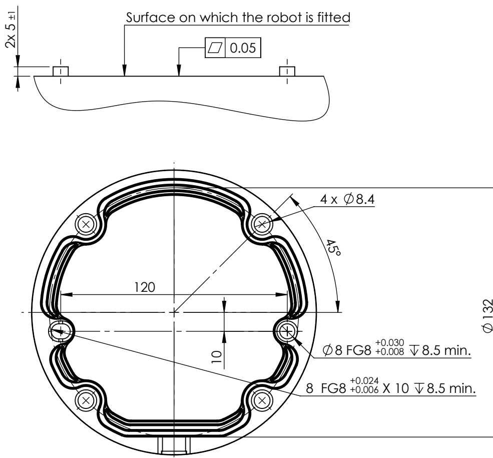
5.1: Odprtine za vgradnjo robota. Uporabite štiri vijake M8 . Vse mere so v mm .
