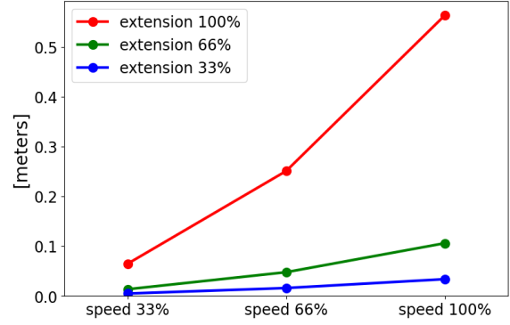
12,5 kg'nin %66'sı için metre cinsinden durdurma mesafesi
