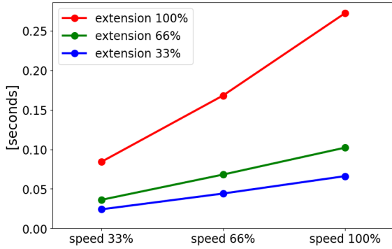
12,5 kg'nin %33'ü için saniye cinsinden durdurma süresi
