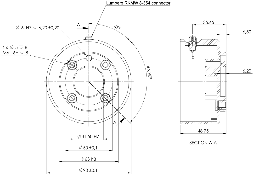
5.2: Aletin çıkış flanşı (ISO 9409-1-50-4-M6), aletin robotun ucuna takıldığı yerdir. Bütün ölçümler mm cinsindendir.
