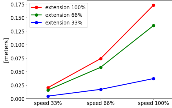
12 kg'lık maksimum taşıma kapasitesi için metre cinsinden durdurma mesafesi
