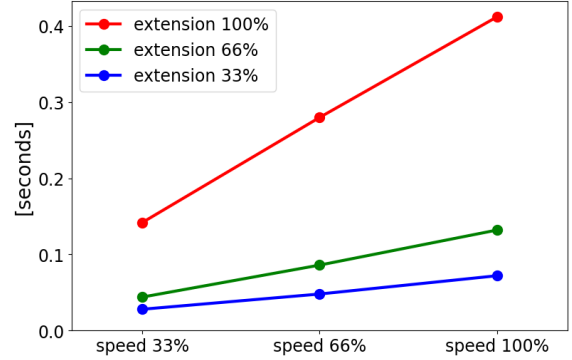
12,5 kg'nin %66'sı için saniye cinsinden durdurma süresi
