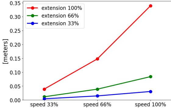
12,5 kg'nin %33'ü için metre cinsinden durdurma mesafesi
