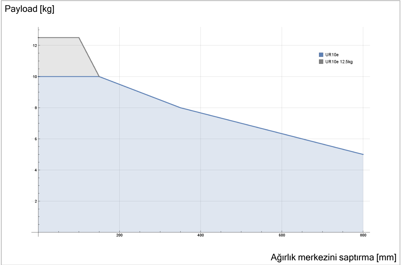
5.3: Nominal taşıma kapasitesiyle ağırlık merkezini saptırma arasındaki ilişki.
