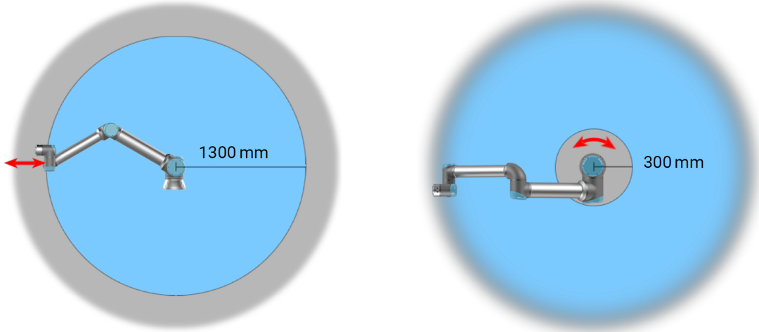
4.1: Robot kolunun fiziksel özelliklerinden dolayı, bazı çalışma alanlarına sıkıştırma tehlikeleriyle ilgili olarak dikkat edilmesi gerekir. Bilek 1 eklemiyle robot tabanı arasında en az 1300 mm olduğunda, radyal hareketler için bir alan (sol) tanımlanır. Diğer (sağdaki) alan, teğet hareket ederken robotun tabanının 300 mm yakınındadır.
