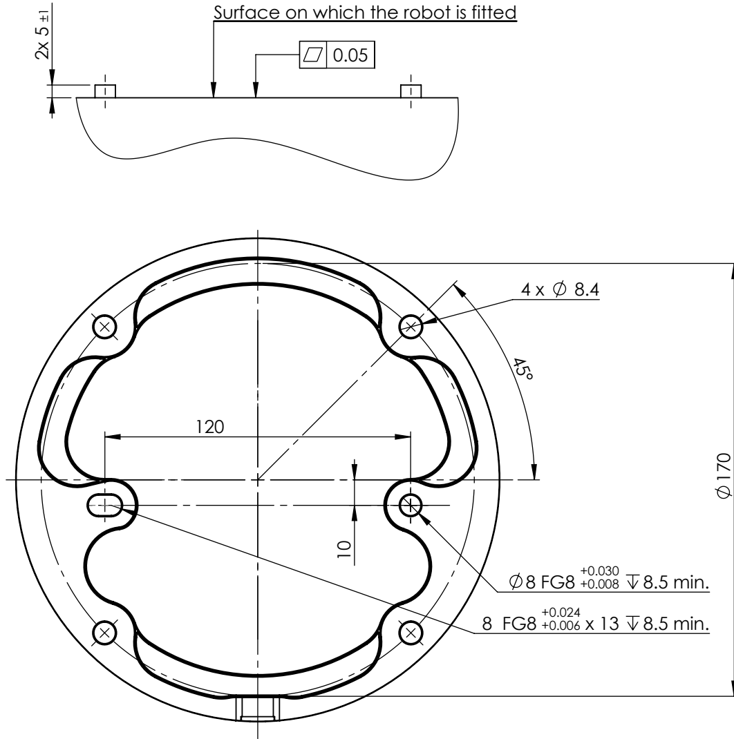
5.1: Robotun montaj delikleri. Dört M8 cıvata kullanın. Bütün ölçüler mm cinsindendir.
