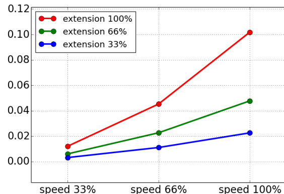
Stopafstand in meters bij 66% van 16 kg
