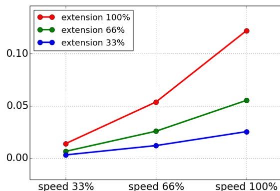
Stopafstand in meters bij de maximale lading van 16 kg
