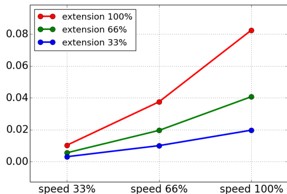
Stopafstand in meters bij 33% van 16 kg
