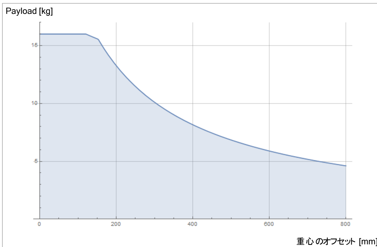
CF :5.1: 定格荷重と重心オフセットとの関係。
