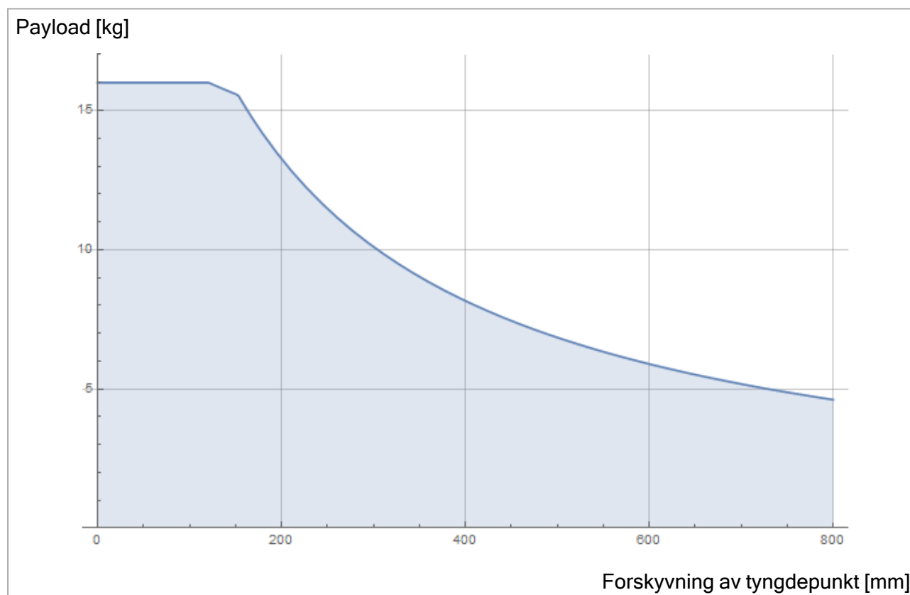
5.3: Forholdet mellom rangert nyttelast og forskyvningen av tyngdepunktet.
