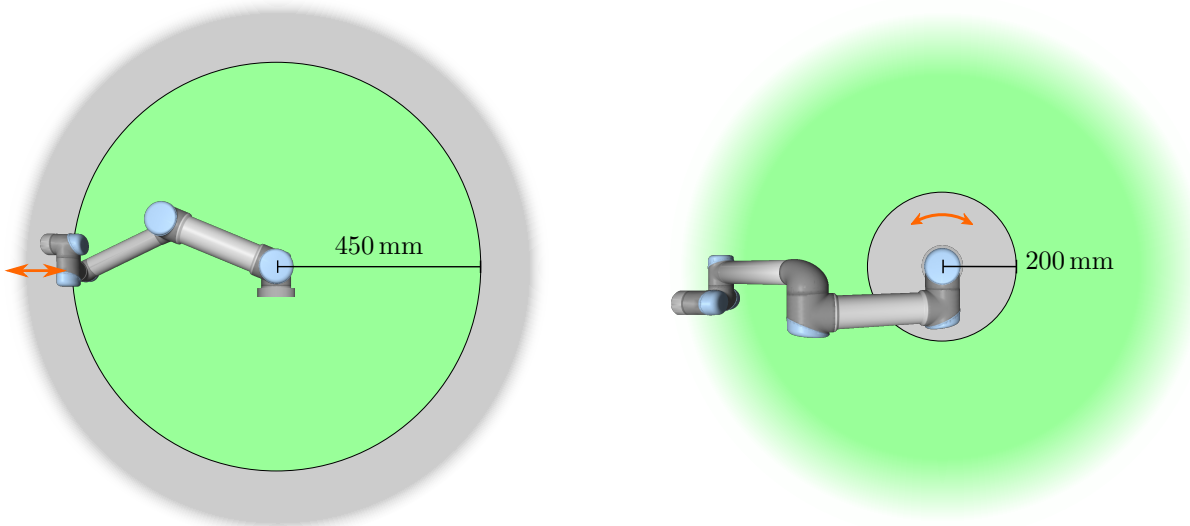
Figure 2.1: 작업영역의 특정 영역은 로봇팔의 물리적 특성 때문에 집히는 위험을 주의해야 한다. 리스트 1 조인트가 로봇베이스로부터 최소한 450 mm 거리인 경우에만 한 영역이 방사형 동작을 위해 정의된다. 접선 방향으로 움직이는 경우, 다른 영역은 로봇베이스로부터 200 mm 거리내에 있다.
