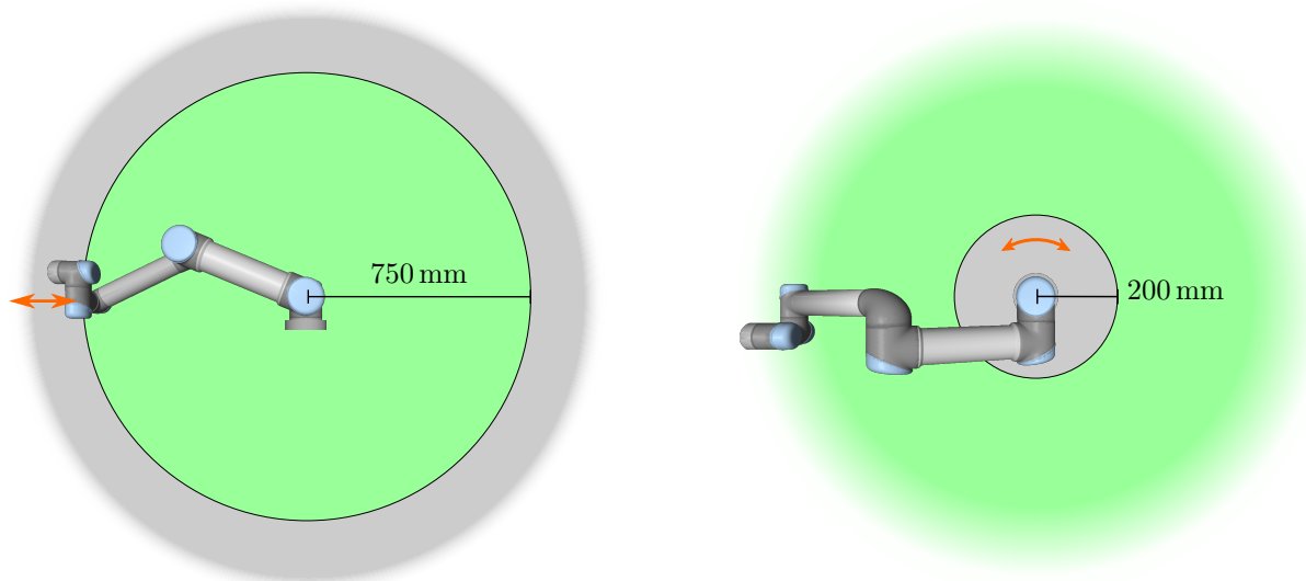
Рис. 2.1: Определенным рабочим зонам должно быть уделено особое внимание в части угроз заземления, связанных с физическими свойствами манипулятора робота. Одна зона отведена под радиальные перемещения, при которых запястье 1 сочленения находится на расстоянии менее 750 мм от основания робота. Другая зона находится в пределах 200 мм от основания робота в случае перемещения по касательной.
