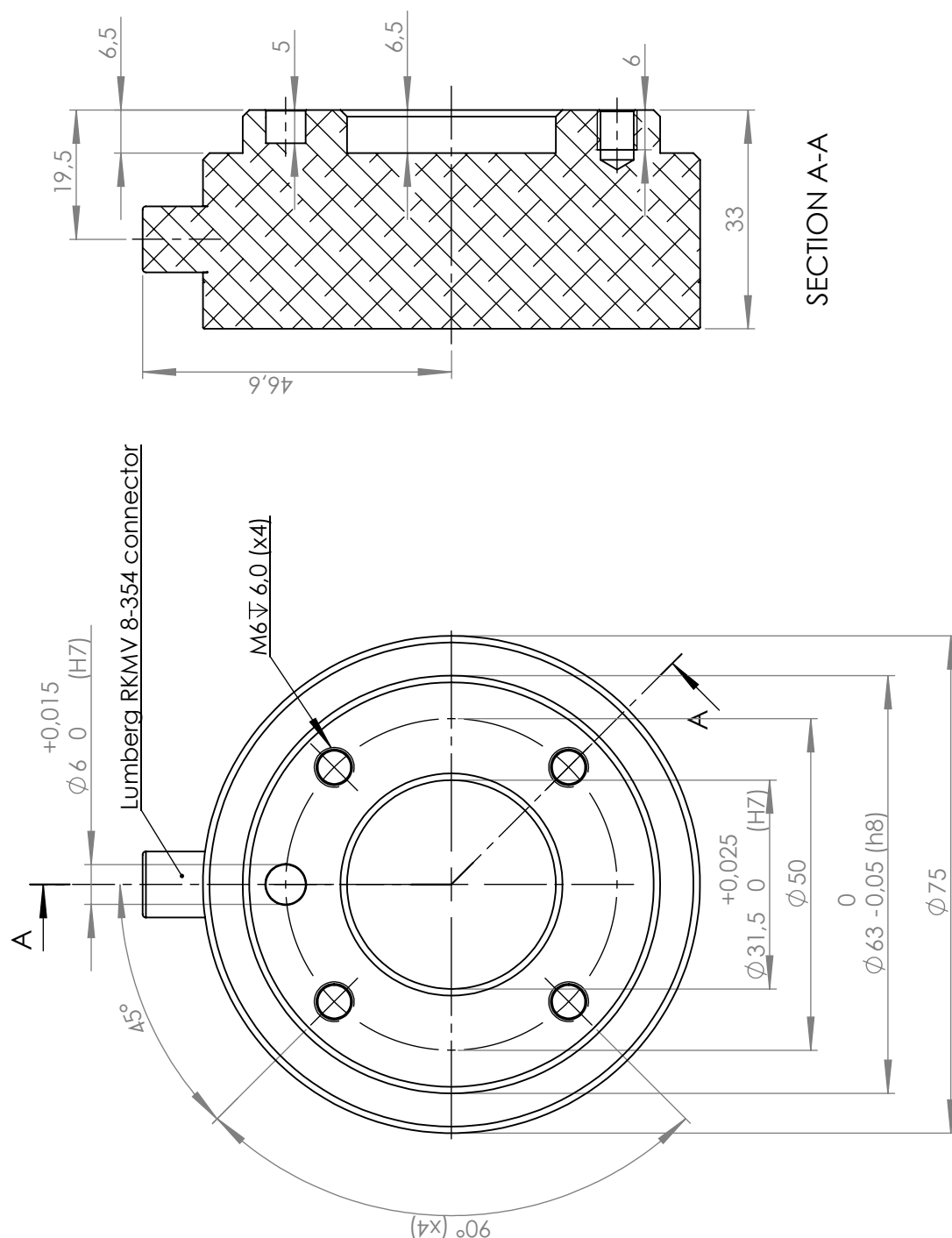
Рис. 4.2: Фланец для подсоединения инструмента, ISO 9409-1-50-4-M6. В этом месте инструмент прикрепляется к наконечнику робота. Все измерения приведены в мм.
